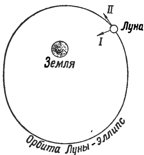
Рис. 2. Вращение Луны вокруг Земли. Стрелка I указывает направление, по которому Луна притягивается Землёй, а стрелка II — направление, по которому двигалась бы Луна, если бы не было всемирного тяготения. Двигаясь вперёд и одновременно притягиваясь к Земле, Луна описывает криволинейный путь
