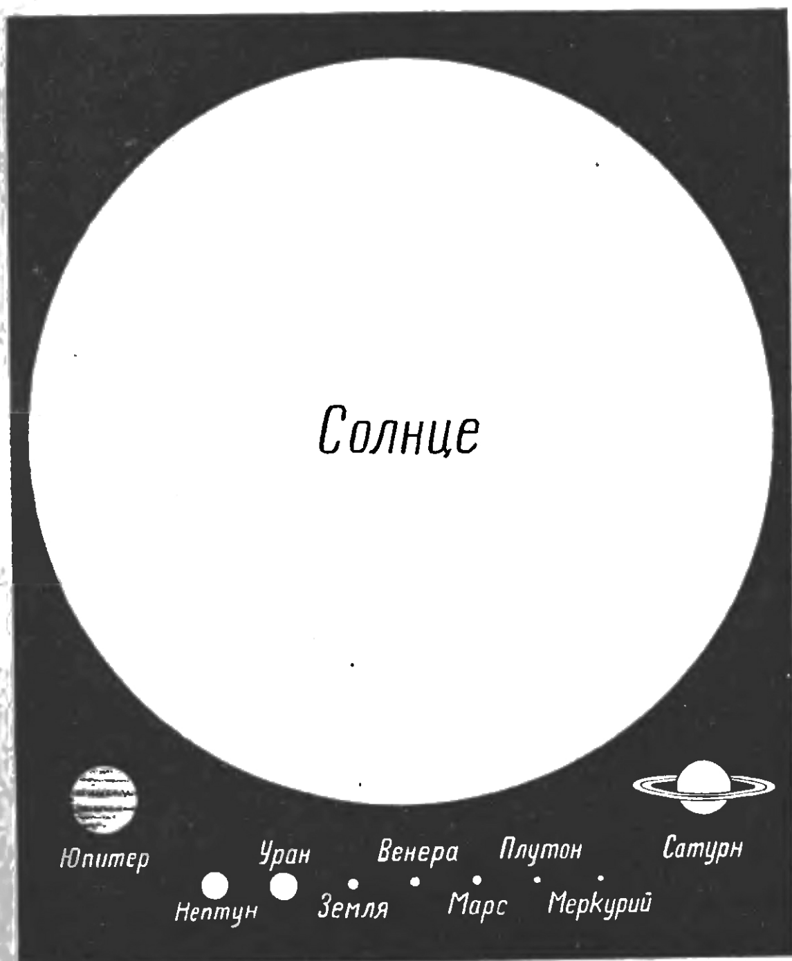
Рис. 5. Сравнительные размеры Солнца и планет
