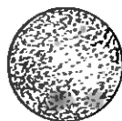
Молодая разреженная звезда желтого цвета
