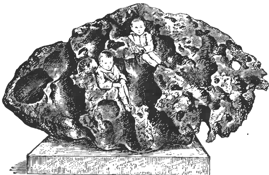
Рис. 3. Один из упавших метеоритов. Для представления об его огромных размерах на нём помещены мальчики
