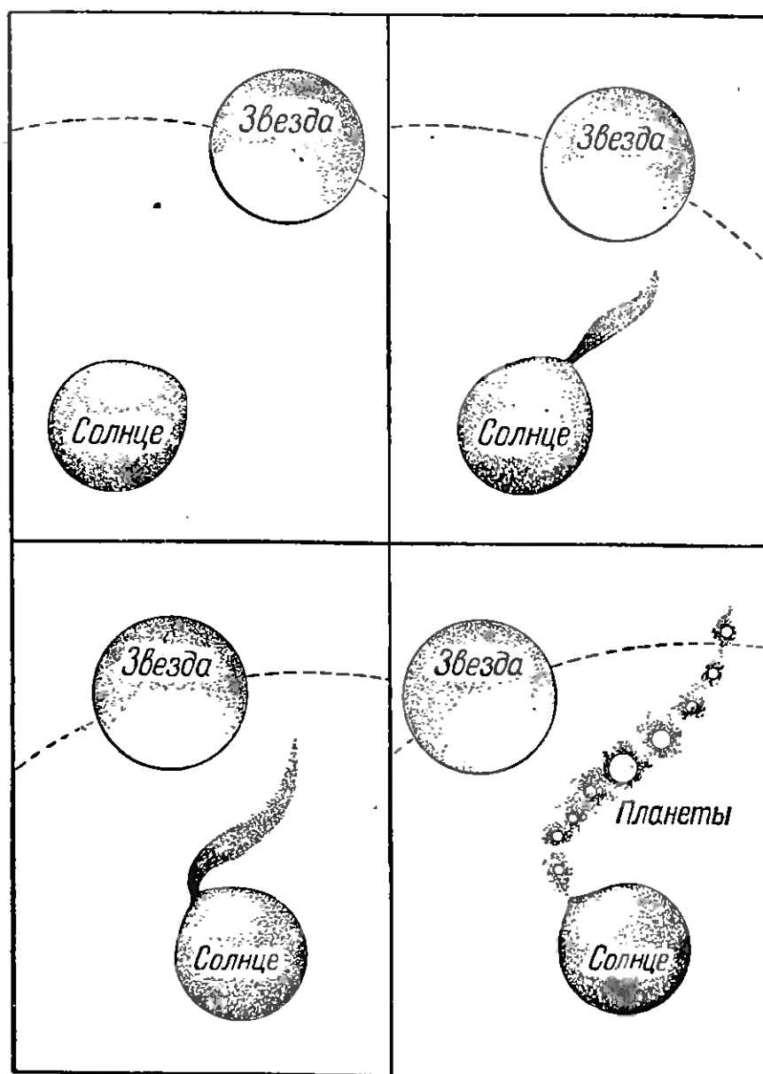
Рис. 14. Так представляют себе учёные рождение планет
