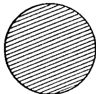
Молодая разреженная холодная звезда красного цвета
