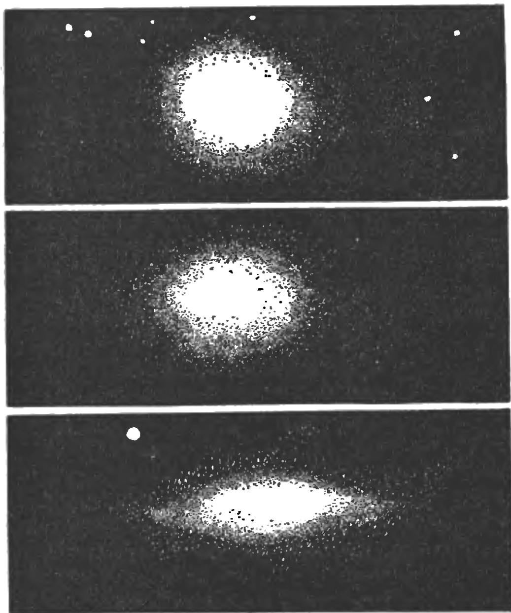
Рис. 11. Такие формы с течением времени принимает большая туманность, прежде чем она превращается в звёздную систему. Вначале она имеет форму шара, а затем сплющивается, напоминая по форме блин
